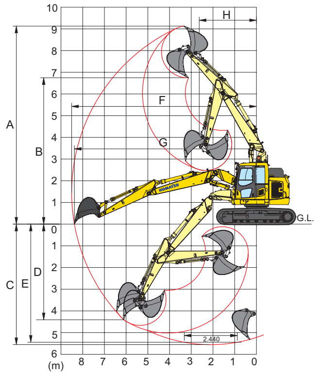
Braccio posizionale
